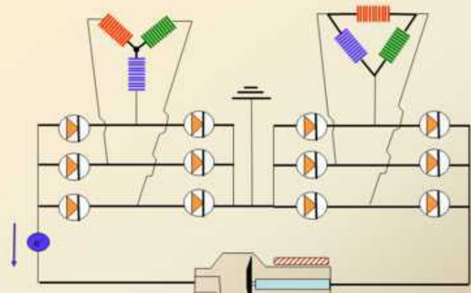
Montage à 12 redresseurs → générateur hexaphasé
