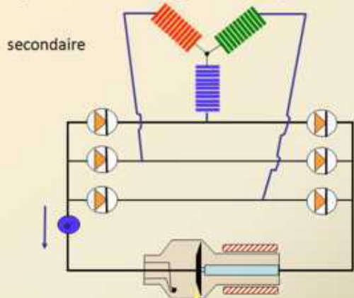
Montage à 6 redresseurs → générateur triphasé
