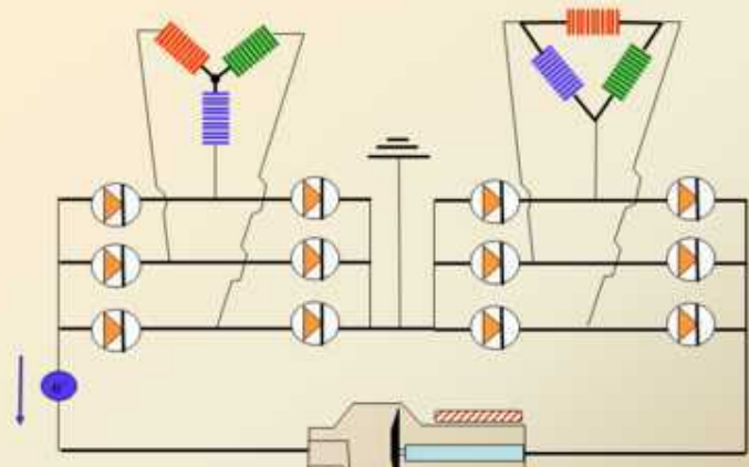
Montage à 12 redresseurs → générateur hexaphasé
