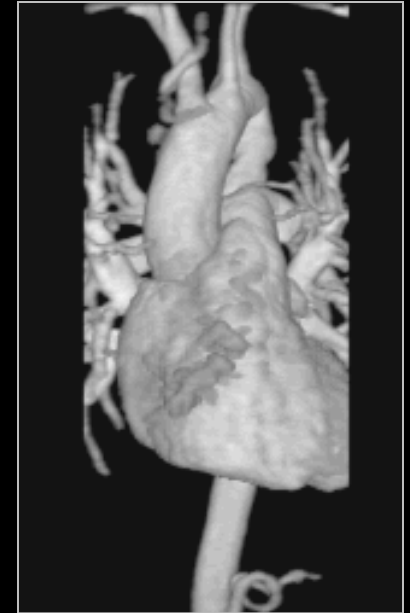
3D Gad-DTPA
