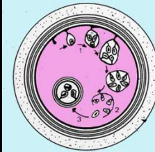
E. granulosus
